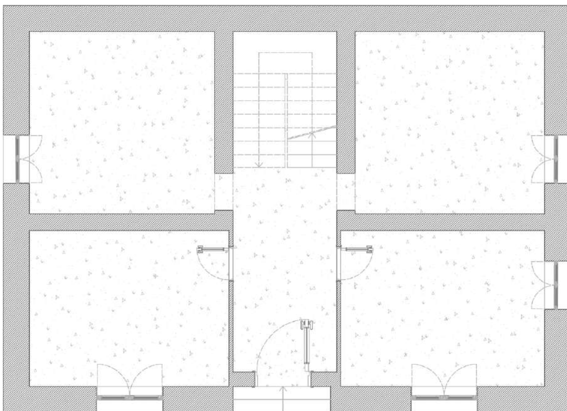
PIANTA PIANO TERRA PIANTA NON IN SCALA PiuValoreCasa.com
